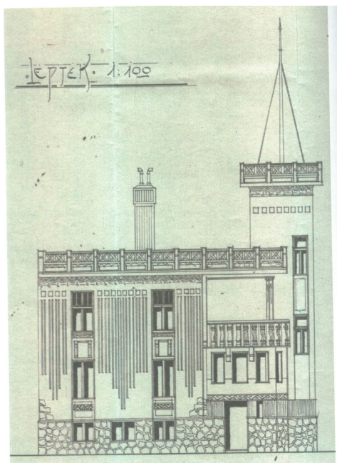
A Hübschl-villa homlokzati rajza 1909-ből (PML) The facade drawing of the Hübschl villa from 1909 (PML) Zeichnung über die Fassade der Hübschl-Villa aus 1909 (PML)
