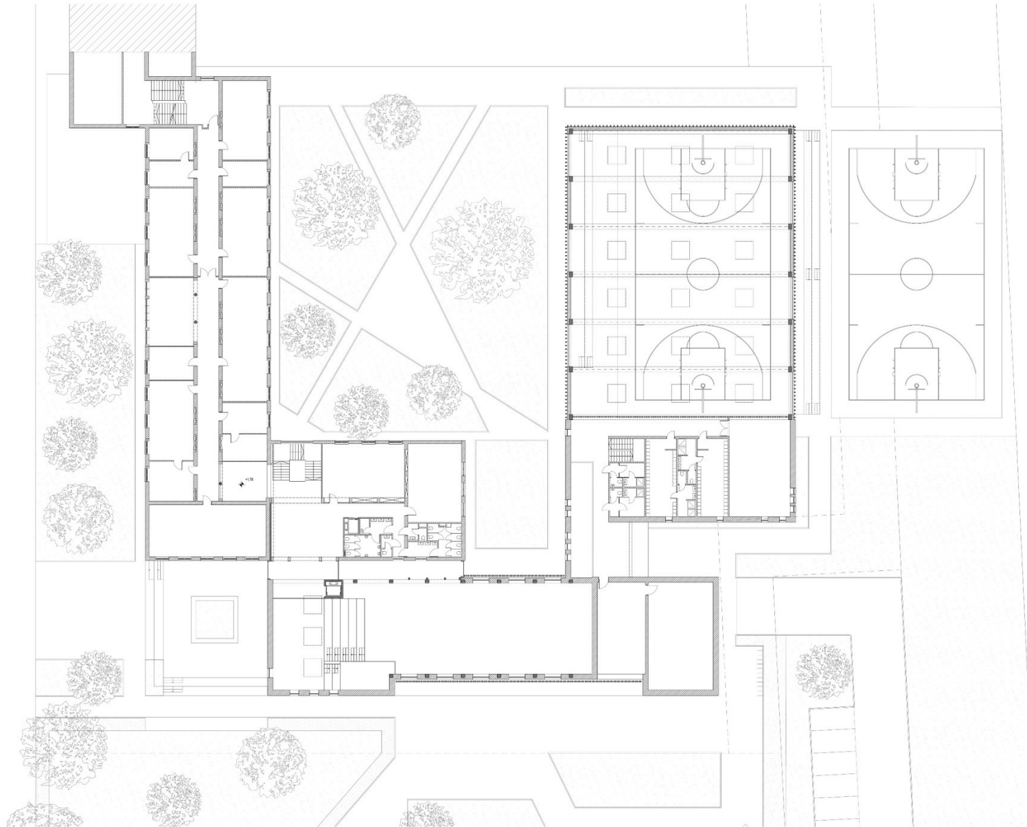
I. EMELETI ALAPRAJZ
