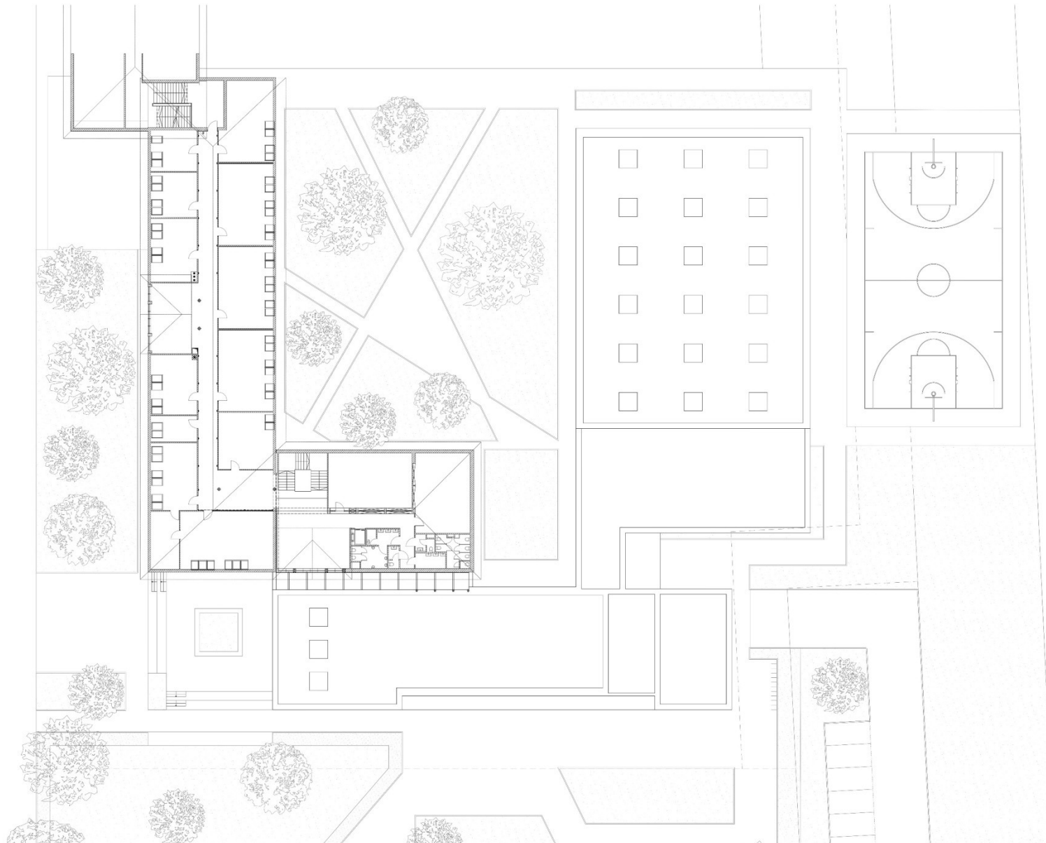
TETŐTÉRI ALAPRAJZ
