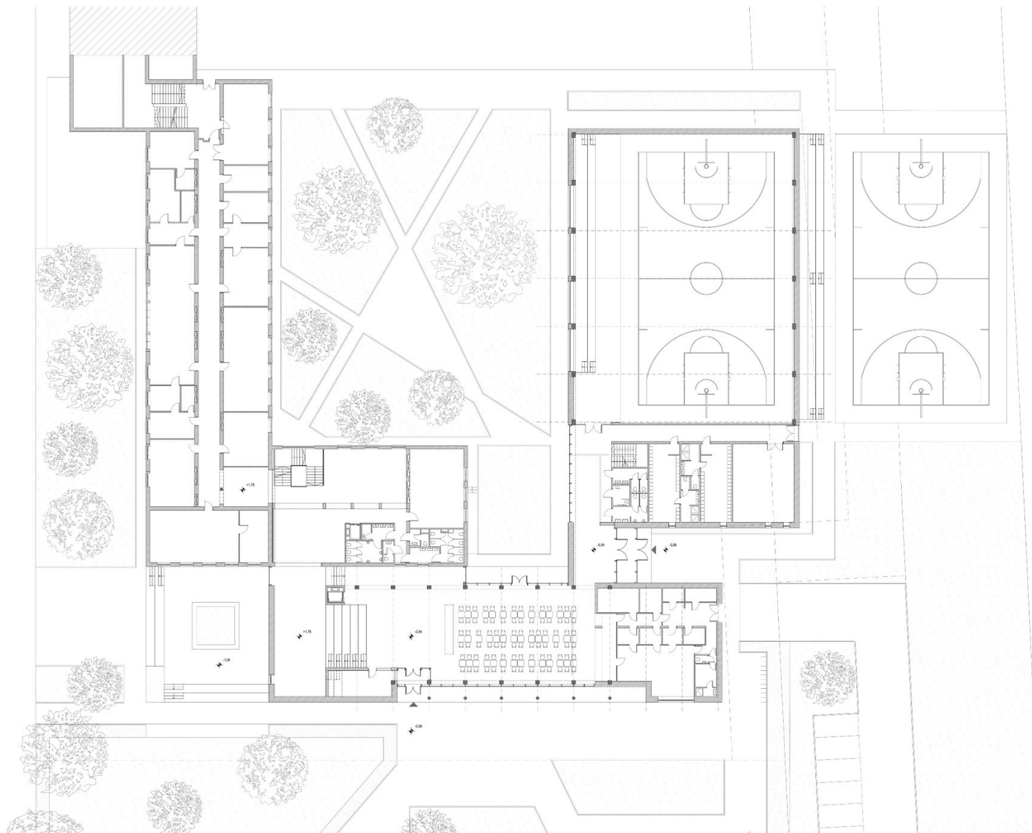
FÖLDSZINTI ALAPRAJZ
