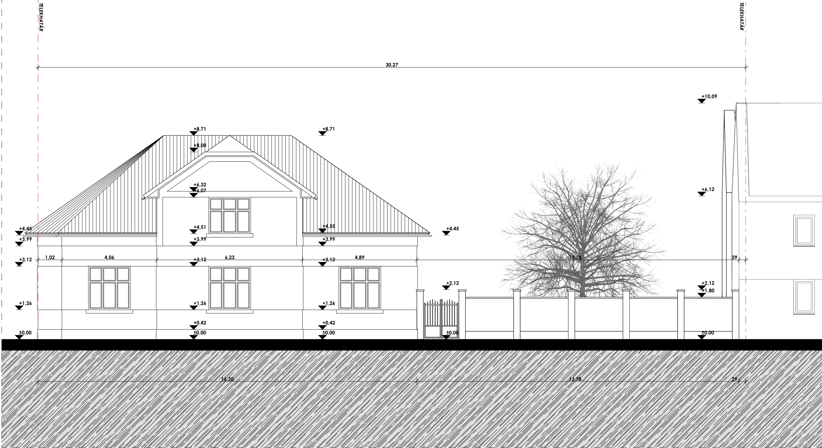
Meglévő Görgey Artúr utcai homlokzat M 1:100
