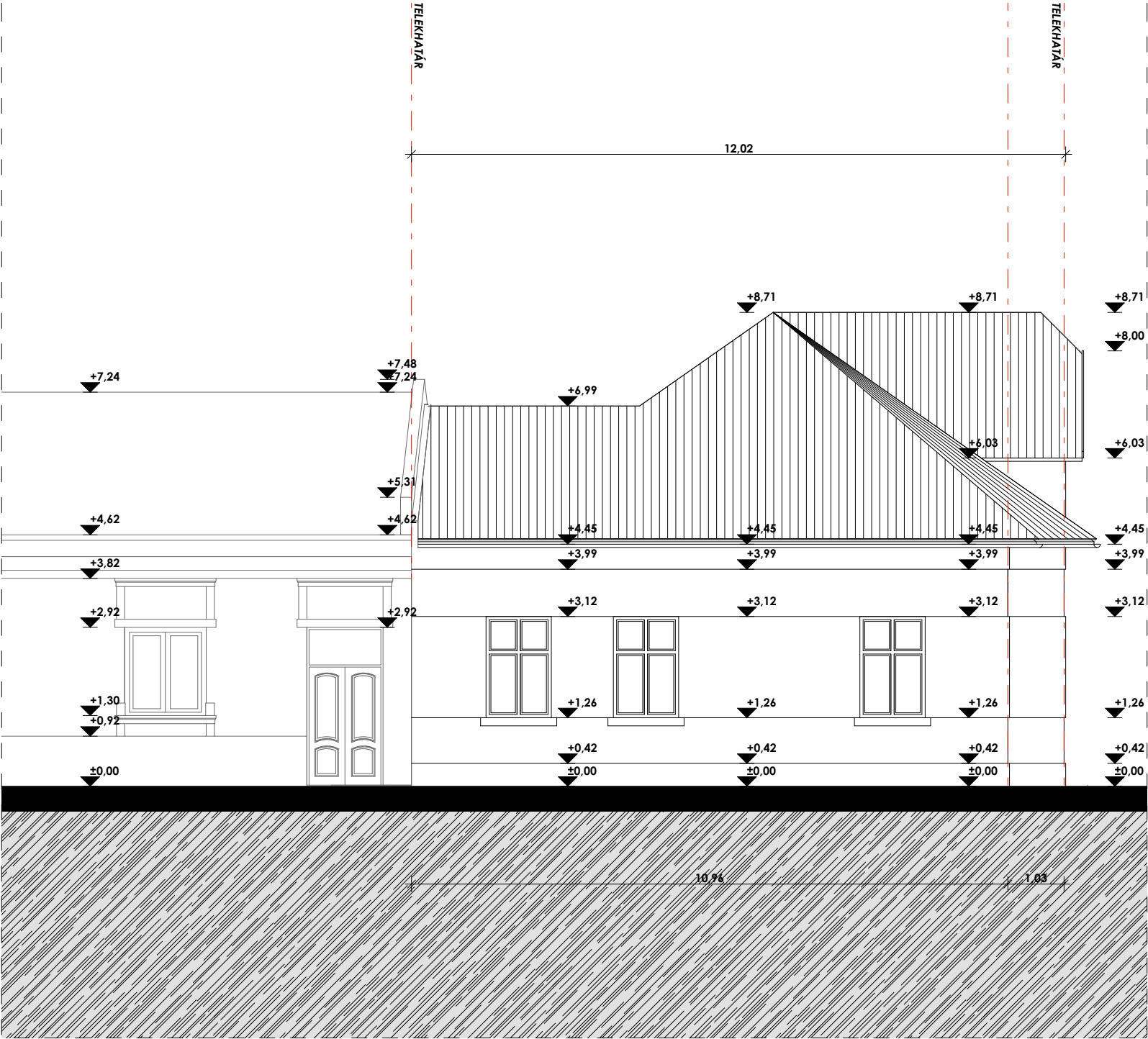
Meglévő Posta park felőli utcai homlokzat M 1:100
