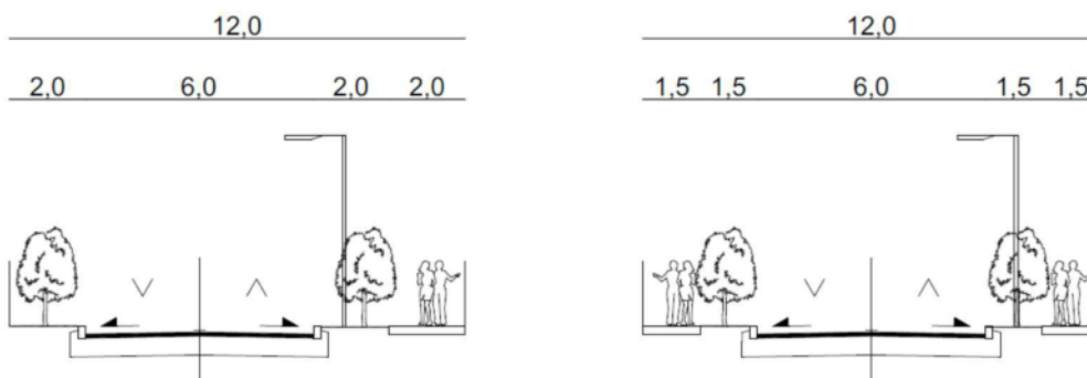
Kiszolgáló út zárt csapadékvíz elvezetéssel
