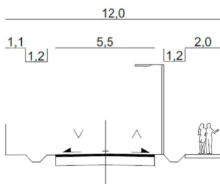
Kiszolgáló út nyílt árokkal
